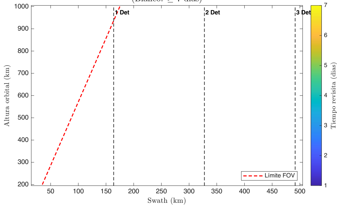
Tiempo Revisita - 2 Satelite(s); 1 Telescopio(s): Refractivo; Detector 2 (Blanco: \geq 7 dias)
